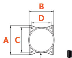
Detalle anclaje
