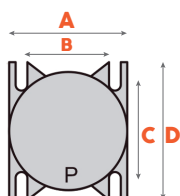
Detalle anclaje
