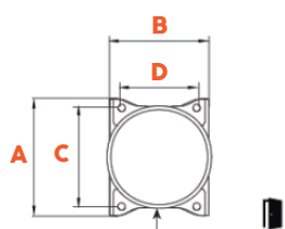
Detalle anclaje
