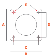
Detalle anclaje
